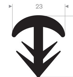
Artikelcode 3921605015 Kwaliteit EPDM Hardheid 70° Shore Kleur Zwart Lengte 25 meter
