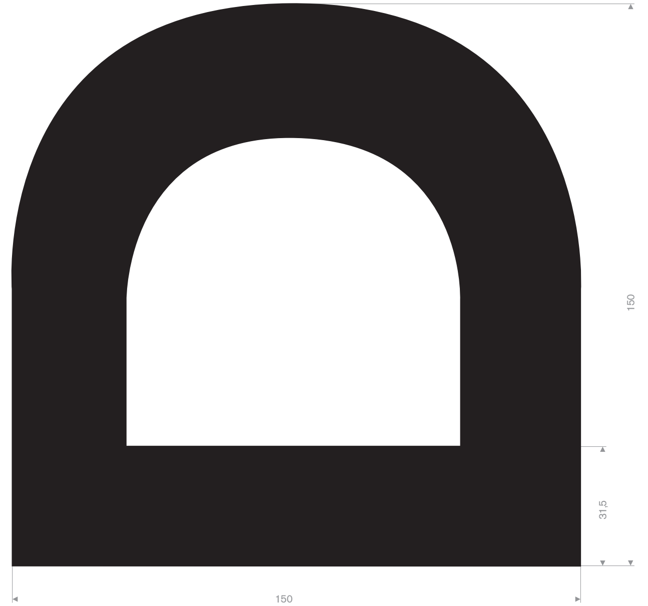
Artikelcode 3921515 015 Kwaliteit EPDM Hardheid 70° Shore Kleur Zwart Lengte 5 meter
