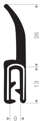
Artikelcode 3924500875 Kwaliteit Volrubber EPDM Klembereik 1,5-4 mm Kleur Zwart Lengte 30 meter
