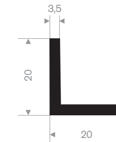
Artikelcode 3921652020 Kwaliteit EPDM Hardheid 70° Shore Kleur Zwart Lengte 50 meter
