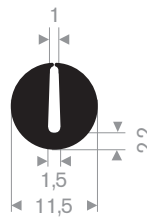
Artikelcode 3921100175 Kwaliteit EPDM Hardheid 70° Shore Kleur Zwart Lengte 100 meter
