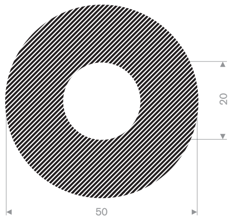
Artikelcode 3048050020 Kwaliteit EPDM Hardheid 15° Shore Kleur Zwart Lengte 15 meter
