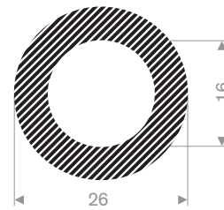
Artikelcode 3048026016 Kwaliteit EPDM Hardheid 15° Shore Kleur Zwart Lengte 50 meter
