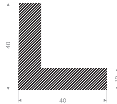
Artikelcode 3922500101 Kwaliteit EPDM Hardheid 15° Shore Kleur Zwart Lengte 25 meter
